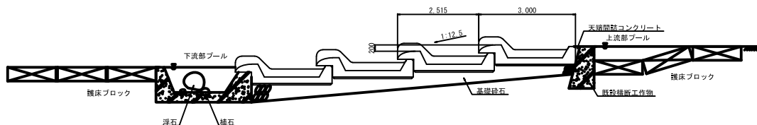
敷設断面図
