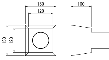
グラウト注入孔詳細図
