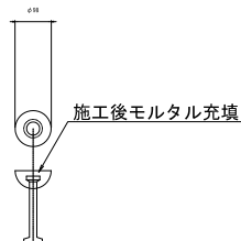
デハアンカー筋詳細図
