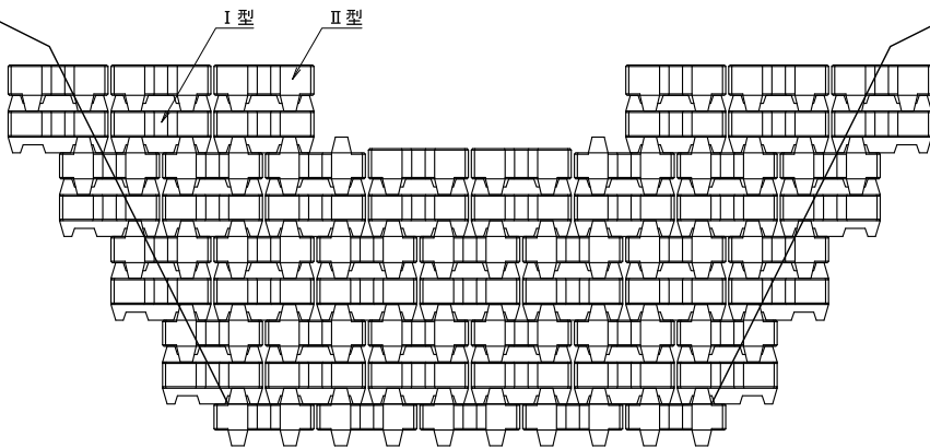
断面図 (A-A)
