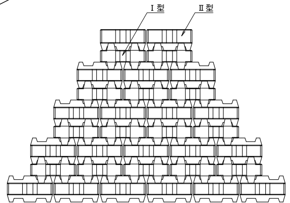
断面図 (B-B)
