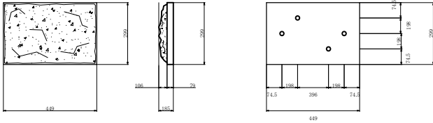
A形 299mm×449mm×70mm 0.134m 2 /枚 約17kg/枚
