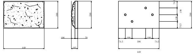
B形 299mm×449mm×70mm 0.134m 2 /枚 約17kg/枚
