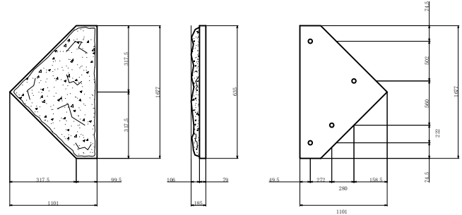
D形 635mm×417mm×70mm 0.164m 2 /枚 約21kg/枚
