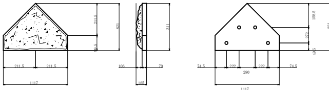
C形 311mm×423mm×70mm 0.087m 2 /枚 約11kg/枚
