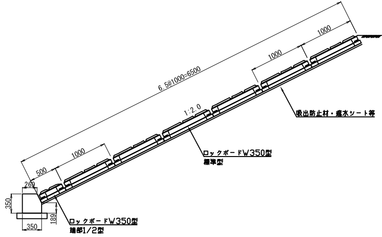
断面図
