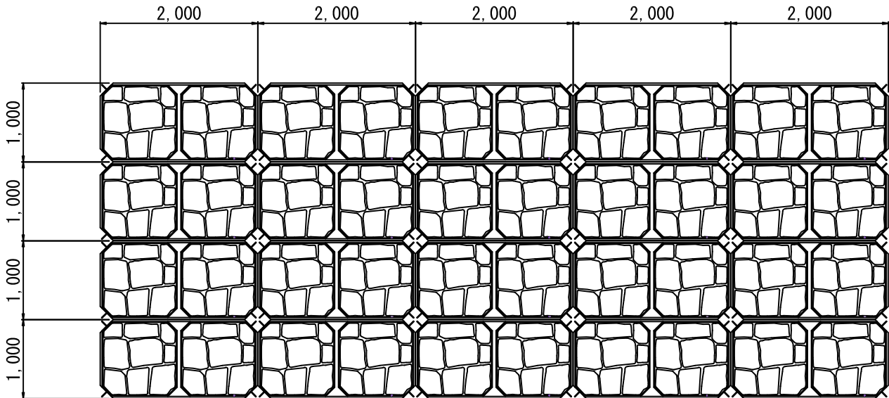
平面図
