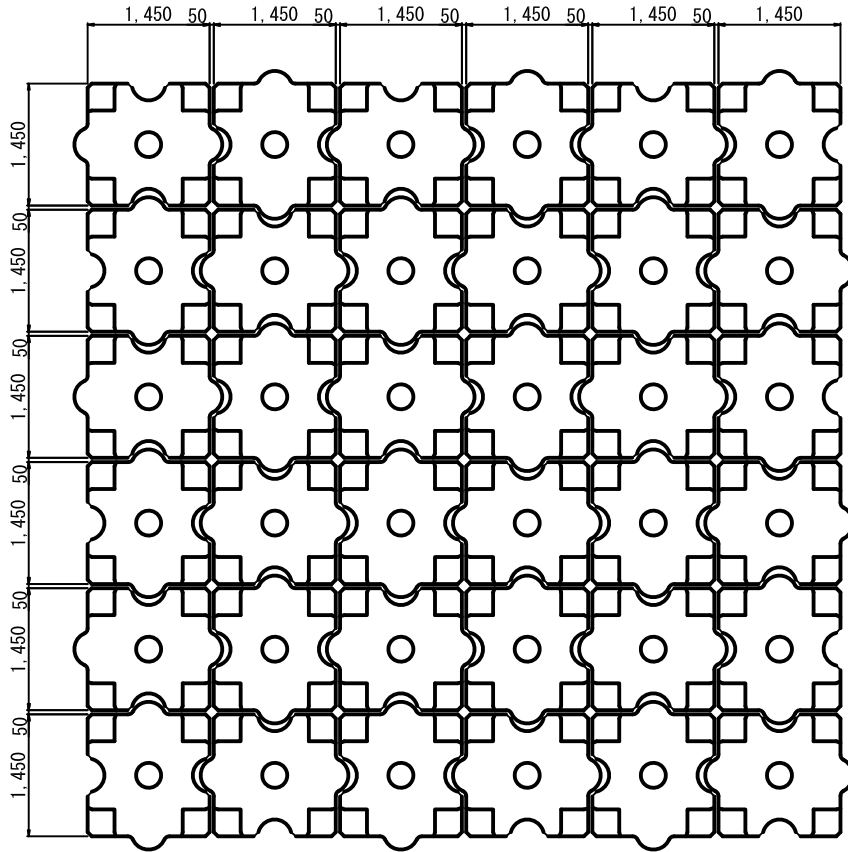
敷設平面図
