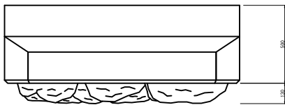
端部型(天端)
