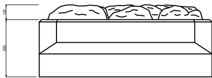
端部型(天端)
