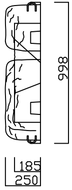
側面図
