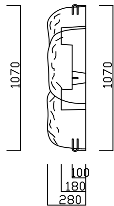
側面図
