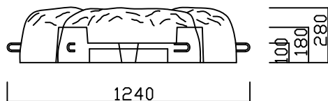
正面図
