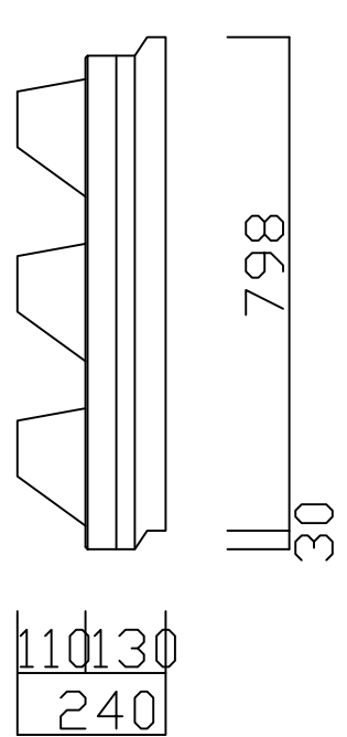
側面図
