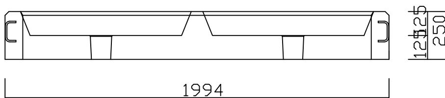
正面図
